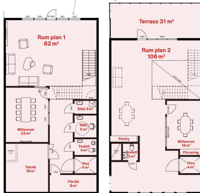
Förslag på gemensamhetsytor i två plan i mitten av fastigheten.
