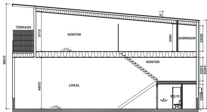
Sektioner A-A, Lokaler
