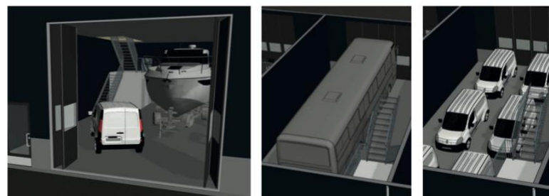
Exempelbilder på förråd/garage och dess användning (17 m djup, 9 m bred och 4,8 m hög). Alla förråd/garage har golvbrunn och kopplad till oljeavskiljare.
