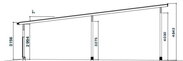
FASAD MOT SYDOST
